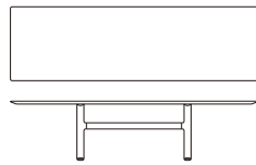
T-386 dining table W3000×D900×H720
