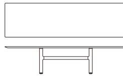
T-387 dining table W3200×D900×H720
